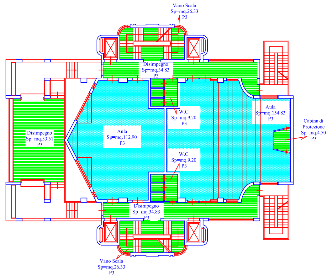
Piano Terzo H=mt.3.70
