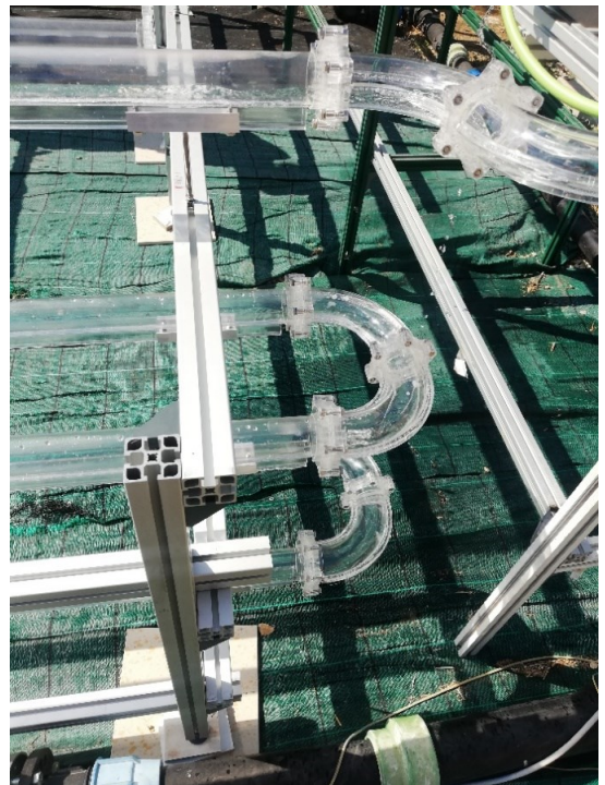
Fig. 4: Particolare su raccordi a U in PMMA
