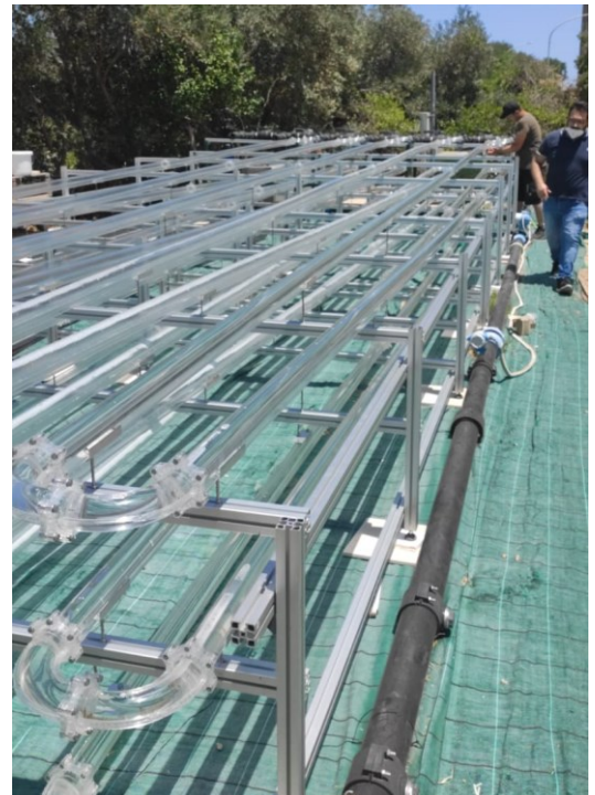
Fig. 2: Vista del fotobioreattore
