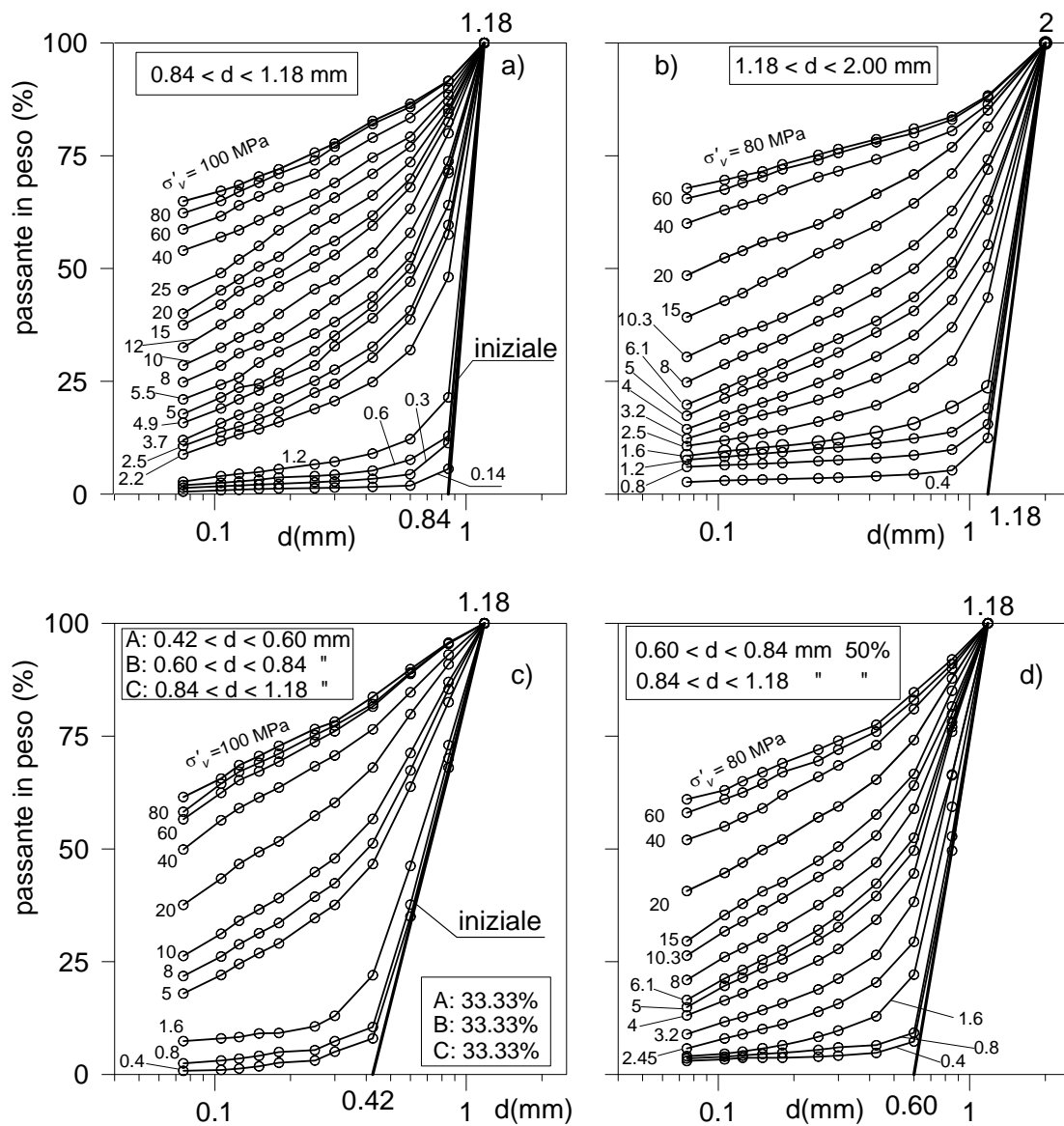
Figura 6. Composizione granulometrica a fine prova delle sabbie 5, 6, 7 e 8 di figura 2. Si noti che a parità di \sigma'_v il crushing è meno intenso nelle sabbie inizialmente più assortite (miscela c) e d)).
