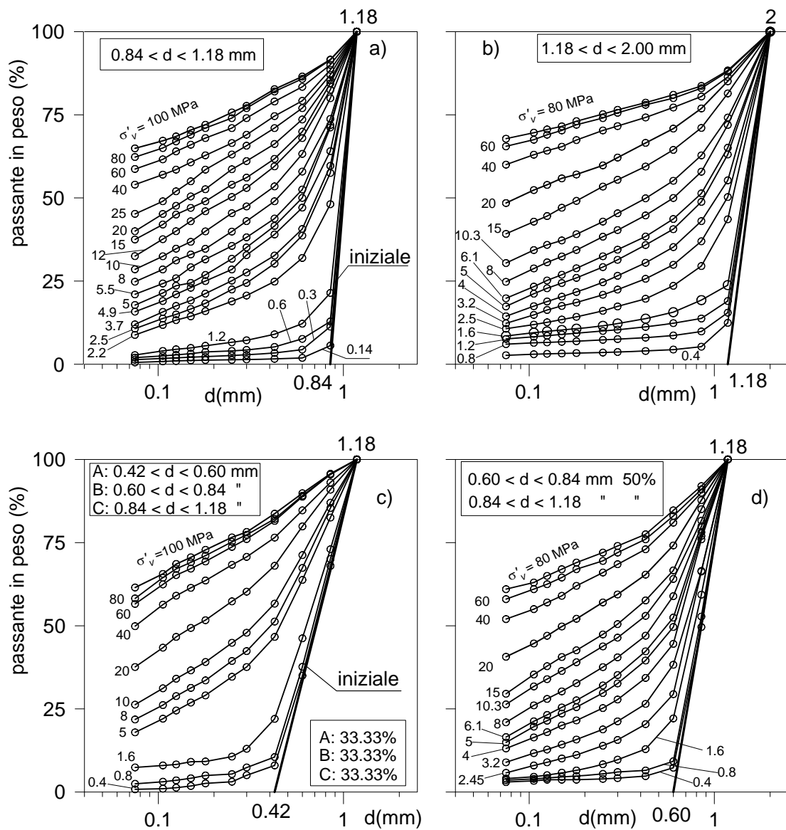
Figura 6. Composizione granulometrica a fine prova delle sabbie 5, 6, 7 e 8 di figura 2. Si noti che a parità di \sigma'_v , il crushing è meno intenso nelle sabbie inizialmente più assortite (miscela c) e d)).
