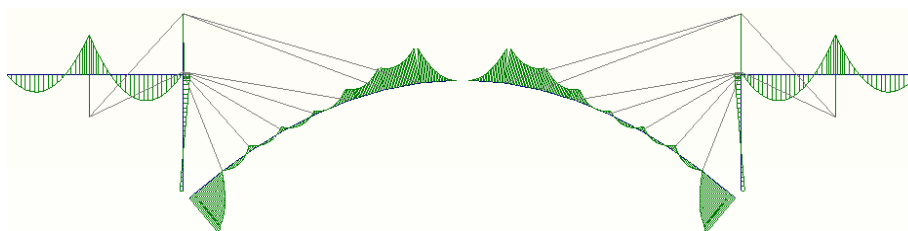
Figura 15.- Diagramma dei momenti flettenti nell'ultima fase a sbalzo.
